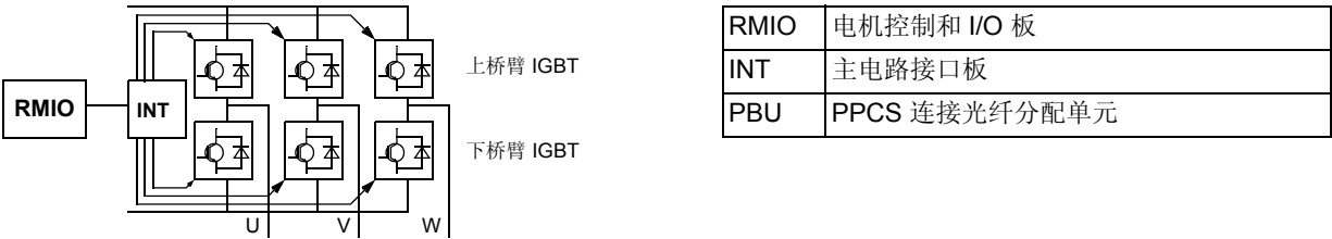
逆变器模块框图 (2 ~ 12 个并联逆变器 )
