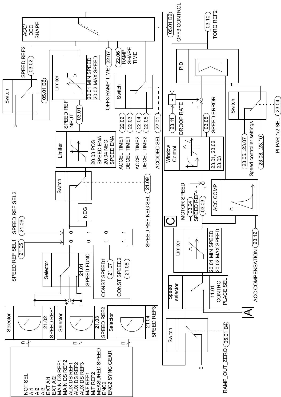
下面的框图表示速度给定链：
