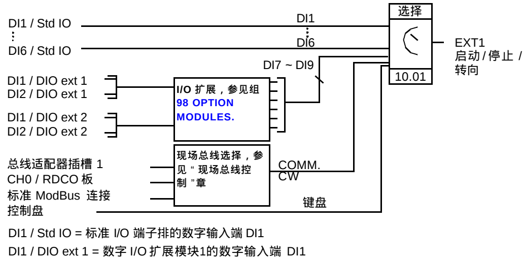
方框图：EXT1 的给定信号
