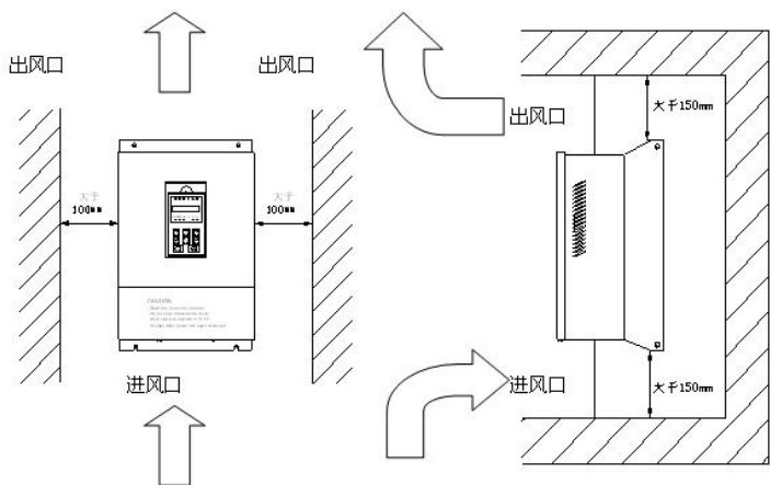
DM 系列变频器的安装空间
