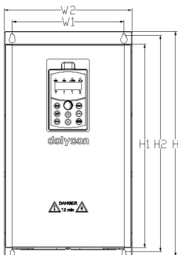
b) 适用于 CT200-4T-15G-B~CT200-4T-110G
