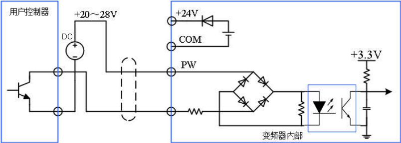
图 3-26 NPN 型灌电流接线方式
