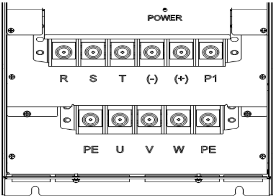
图 3-12 CT200-4T-75G~CT200-4T-110G 主回路接线端子图
