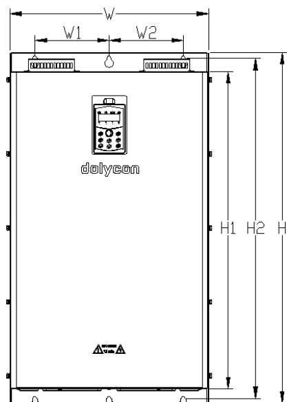
c) 适用于 CT200-4T-132G~CT200-4T-200G
