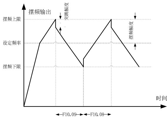
图 6-17 摆频运行
