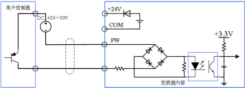
图 3-27 PNP 型拉电流接线方式
