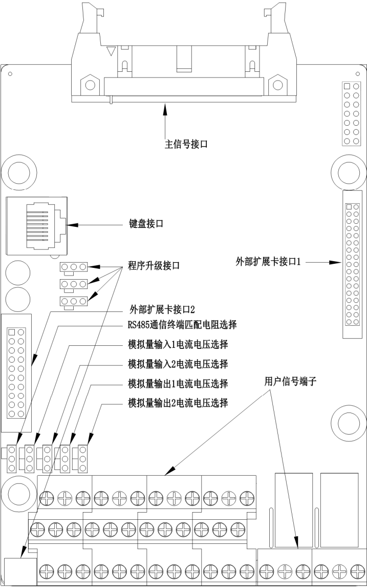
图 3-21 控制板示意图
