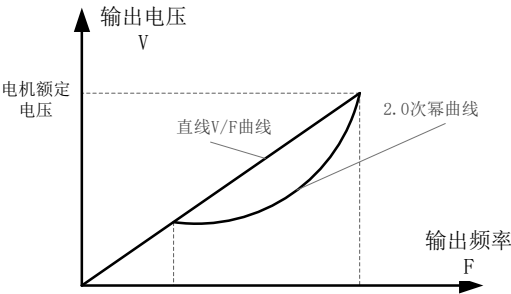
图 6-4 V/F 曲线图
