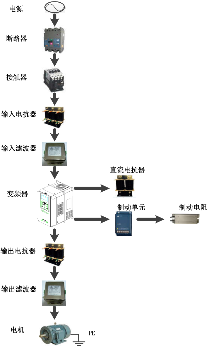
图 3-7 产品外围元器件的标准配置图
