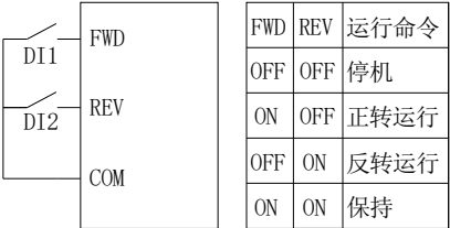
图 6-7 两线式控制 1
