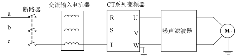
图 3-18 主回路电机侧连接图
