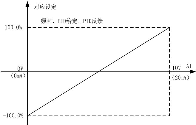
图 6-12 模拟量输入与设定值的对应关系
