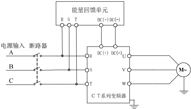
图 3-19 能量回馈单元连接图
