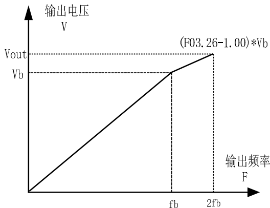
图 6-7 恒功区弱磁系数曲线图
