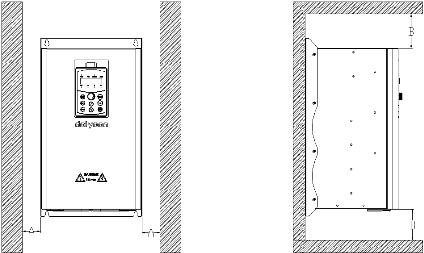
图 3-2 CT200-4T-15G/18.5P-B 及以上功率等级的安装方向和距离要求
