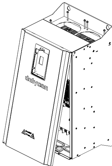
图 3-5 CT200-4T-15G-B 及以上功率 操作面板的安装、拆卸图
