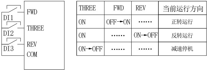
图 6-10 三线式控制 2
