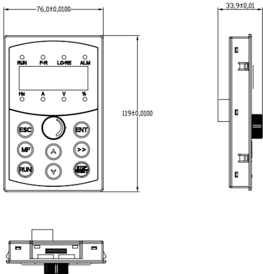
图 2-5 面板外形及尺寸图（单位 mm）
