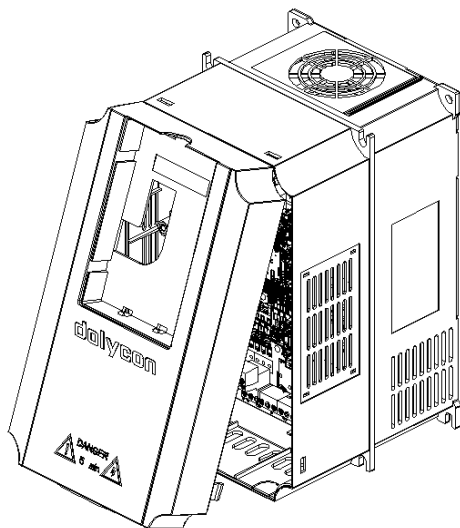
图 ( b ) 拆卸方向
