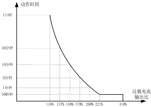
图 6-1 过载保护动作时间与电流比的关系
