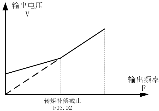
图 6-5 转矩补偿图
