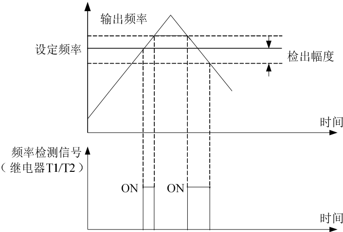
图 6-20 频率到达检测示意图
