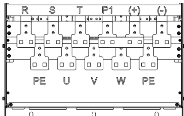
图 3-13 CT200-4T-132G~CT200-4T-200G 主回路接线端子图
