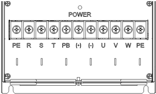
图 3-10 CT200-4T-30G-B~CT200-4T-37G-B 主回路接线端子图
