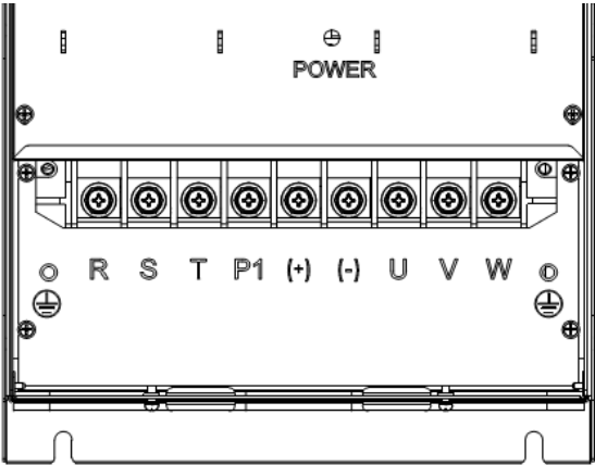
图 3-11 CT200-4T-45G~CT200-4T-55G 主回路接线端子图
