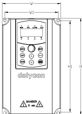
a) 适用于 CT200-2S-2.2G-B 及以下、CT200-4T-11G-B 及以下
