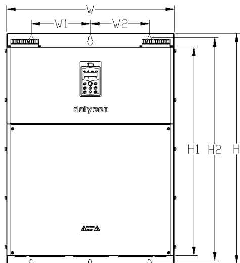
d) 适用于 CT200-4T-220G~CT200-4T-315G
