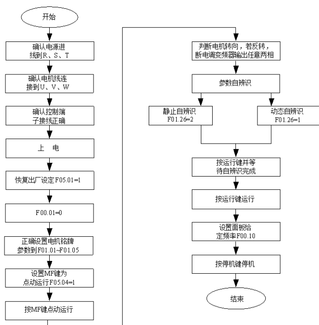
图 4-2 首次上电流程图
