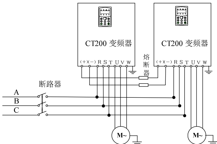
图 3-20 共直流母线的连接
