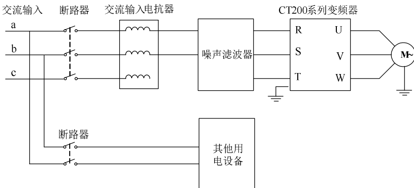
图 3-17 主回路电源侧连接图
