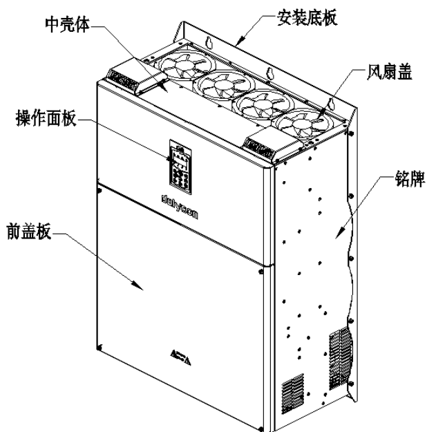
e) CT200-4T-220G~CT200-4T-315G (C8 机箱)
