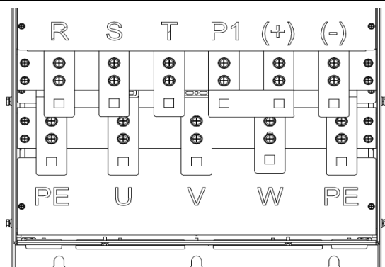
图 3-13 CT200-4T-132G~CT200-4T-200G 主回路接线端子图
