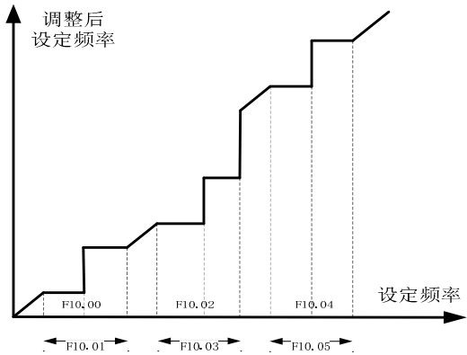
图 6-16 跳跃频率处理
