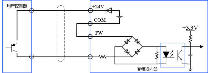
图 3-25 PNP 型拉电流接线方式
