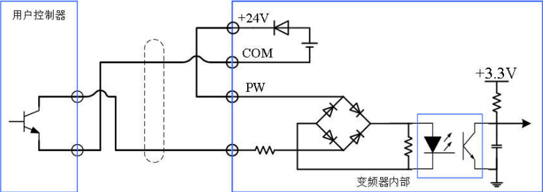
图 3-24 NPN 型灌电流接线方式
