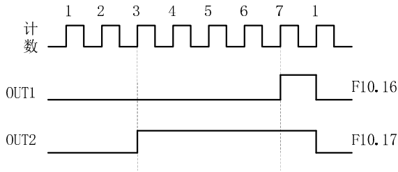
图 6-18 指定计数值与预置计数值
