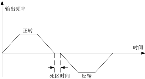
图 6-3 正反转死区时间示意图
