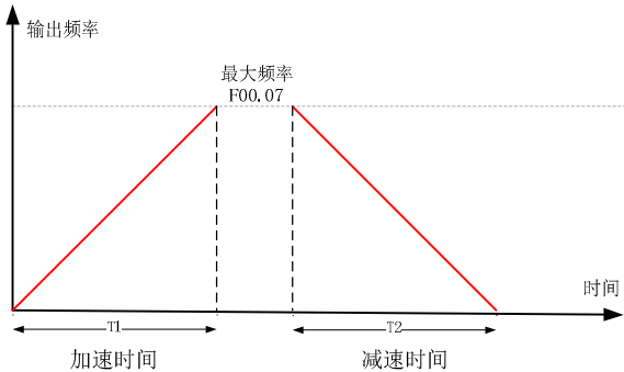
图 6-2 恒加减速曲线图
