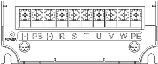
图 3-8 CT200-2S-2.2G-B、CT200-4T-11G/15P-B 及以下功率主回路接线端子图
