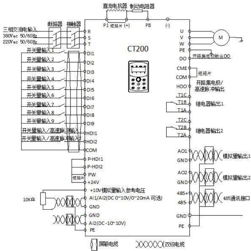
图 3-16 标准接线图
