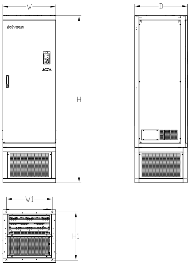
e) 适用于 CT200-4T-350G~CT200-4T-500G
