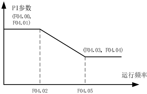
图 6-8 PI 参数与运行频率关系图
