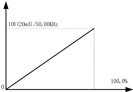
图 6-12 模拟量与高速脉冲输出对应关系
