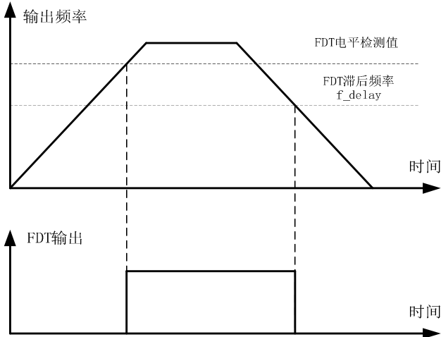
图 6-19 输出频率与 FDT 输出关系图
