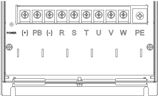
图 3-9 CT200-4T-15G-B~CT200-4T-22G-B 主回路接线端子图
