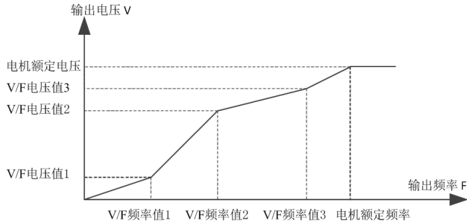
图 6-6 多点 V/F 曲线图
