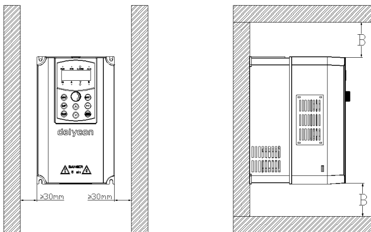
图 3-1 CT200-4T-11G/15P-B 及以下功率等级的安装方向和距离要求
