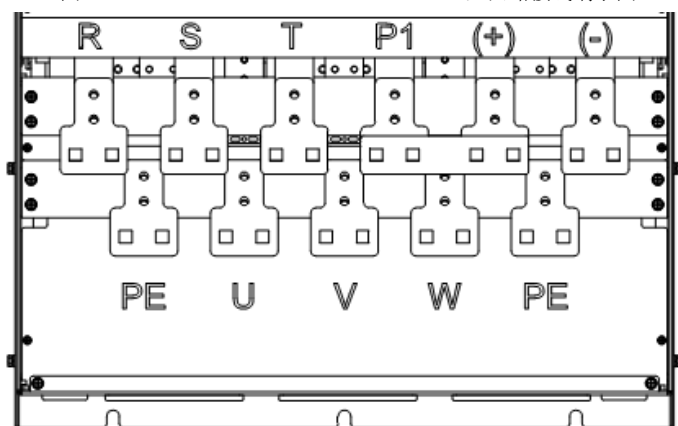
图 3-15 CT200-4T-350G~CT200-4T-500G 主回路接线端子图
