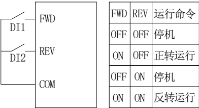
图 6-8 两线式控制 2
