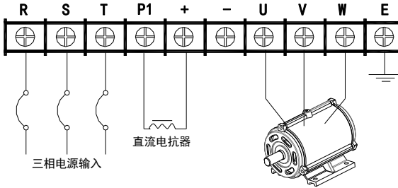
f) 90KW-110KW 变频器主回路端子台配线图 (如图 3-3f)
