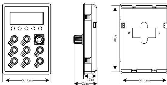
图 2-6 键盘操作器外形及安装尺寸图（11KW 以下）
