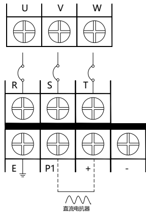
h) 350KW-630KW 变频器主回路端子台配线图（如图 3-3h）
