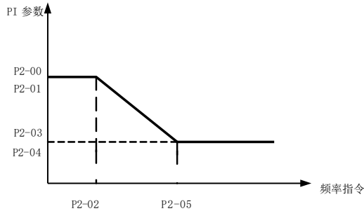
图 6-4 PI 参数示意图
