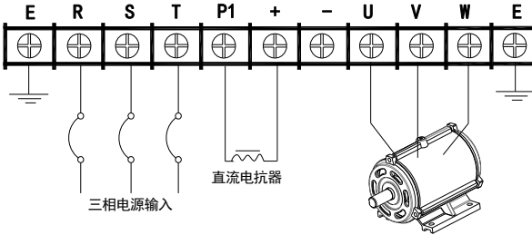
g) 132KW-315KW 变频器主回路端子台配线图 (如图 3-3g)
