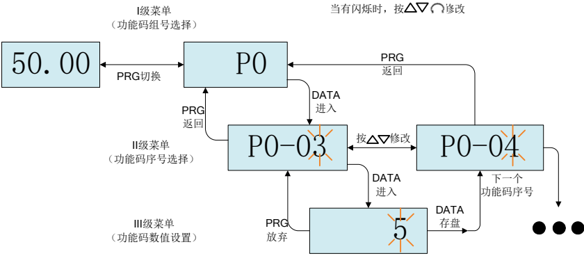
图 4-2 三级菜单操作流程
