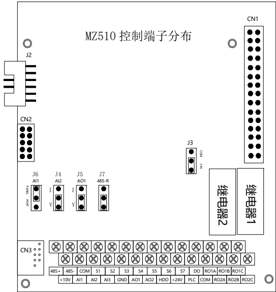
图 3-6 控制端子分布图
