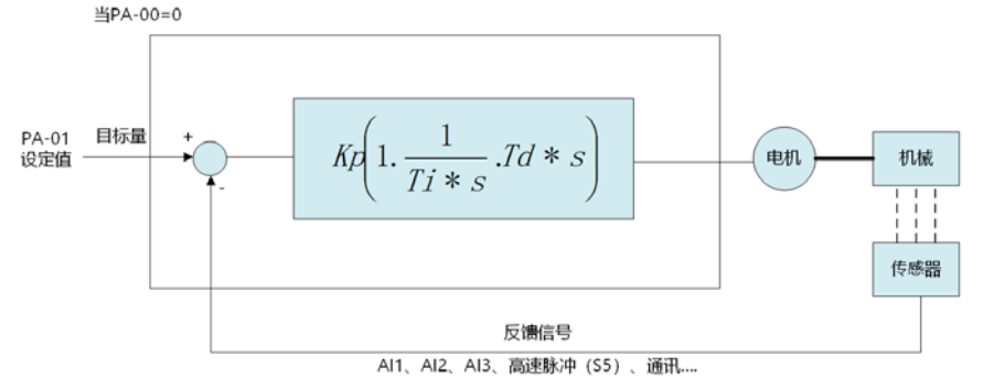
图 6-25 过程 PID 原理框图
