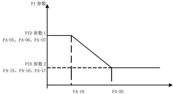
图 6-26 PID 参数切换
