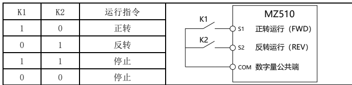
图 6-8 两线式模式 1
