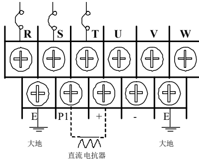
g) 132KW-315KW 变频器主回路端子台配线图 (如图 3-3g)
