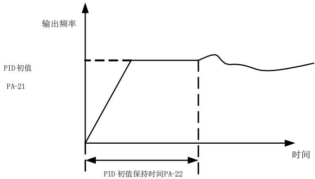
图 6-27 PID 初值的功能示意图
