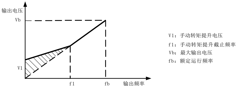
图 6-5 手动转矩提升示意图
