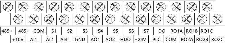
图3-4 控制回路接线端子图
