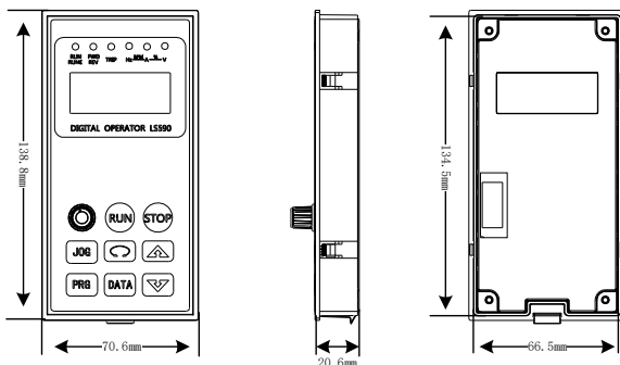
图 2-5 键盘操作器外形及安装尺寸图（11KW（含）以上）
