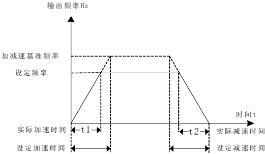
图 6-3 加减速时间示意图
