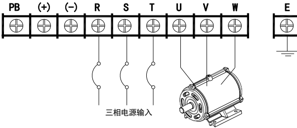
e) 55KW-75KW 变频器主回路端子台配线图 (如图 3-3e)
