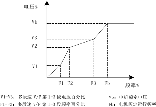
图 6-6 多点 V/F 曲线设定示意图
