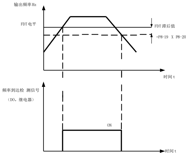
图 6-16 FDT 电平示意图
