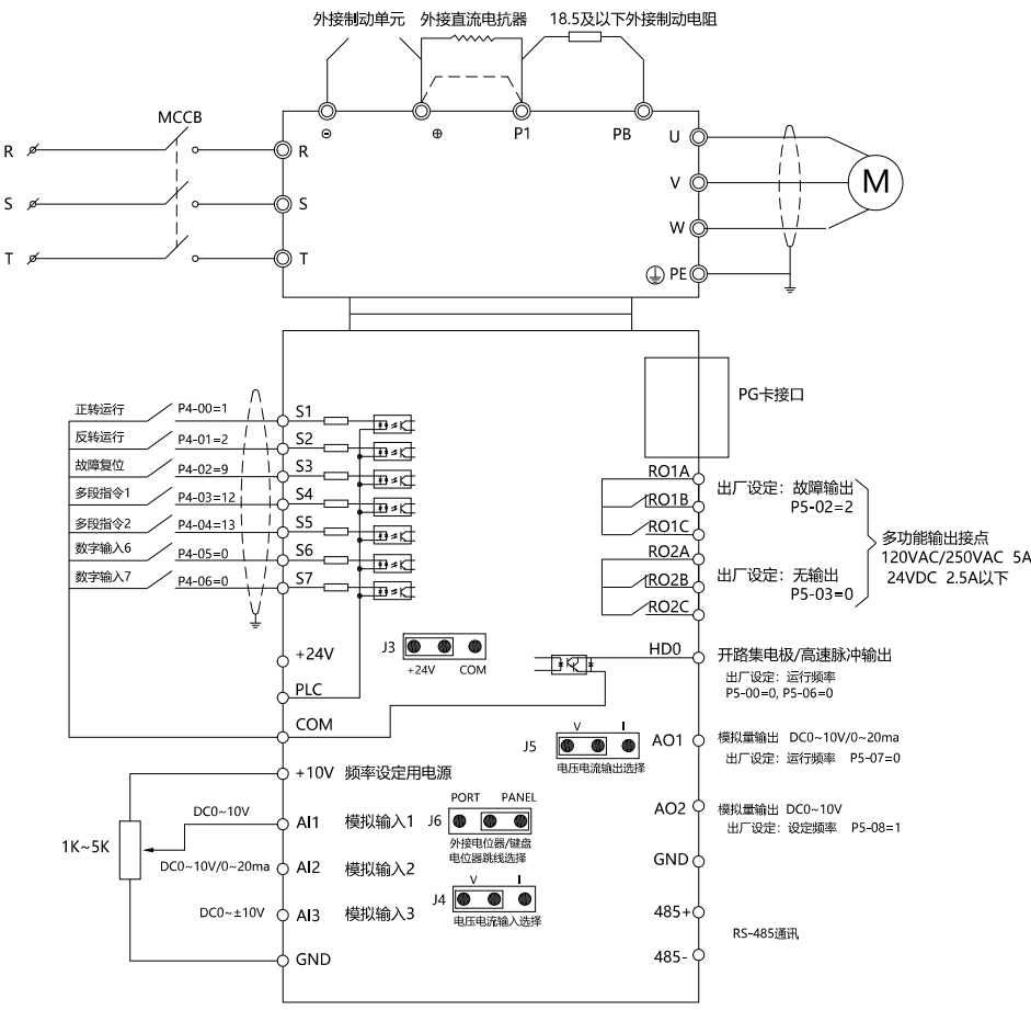
图 3-5 标准接线图
