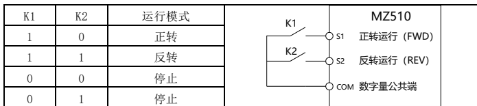
图 6-9 两线式模式 2
