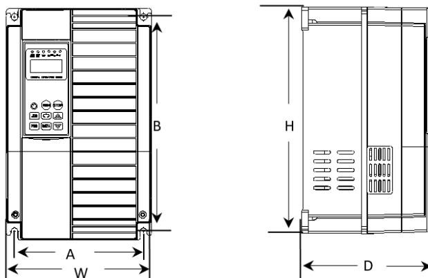
图 2-4 变频器外形尺寸示意图
