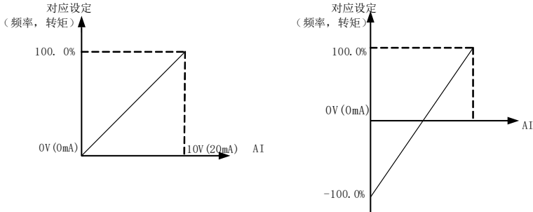
图 6-12 模拟给定与设定量的对应关系
