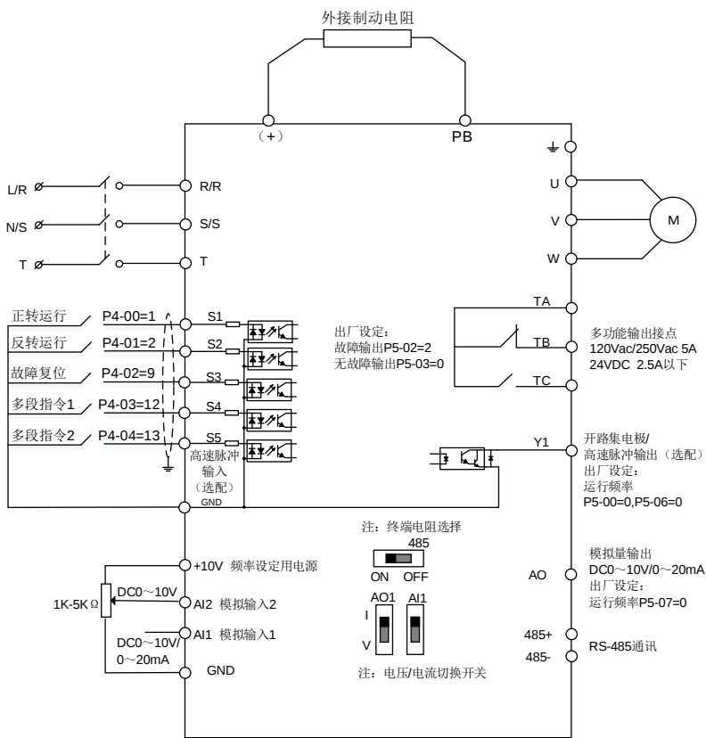
图 3-4 标准接线图
