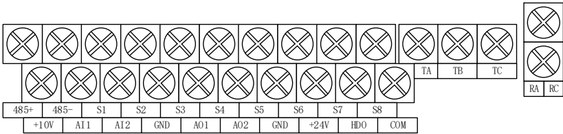
图 3-5 控制回路接线端子图
