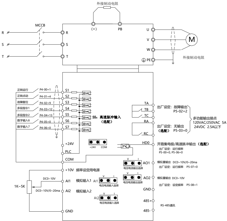
图 3-6 标准接线图
