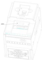
EM60-485 安装方式
