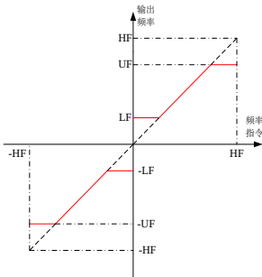
HF：最高频率 UF：上限频率 LF：下限频率
