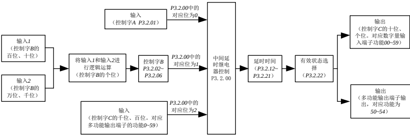
中间延时继电器控制字 B 的控制逻辑功能说明
