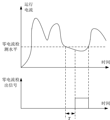
T为零电流检测延迟时间
