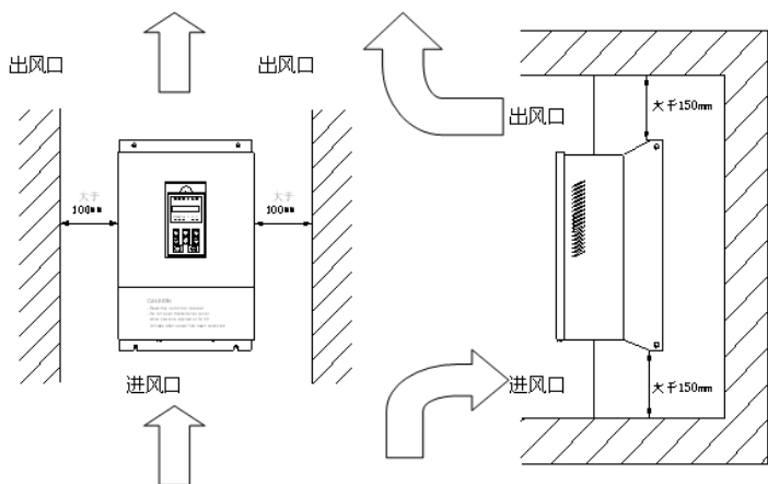
EM60 系列变频器的安装空间
