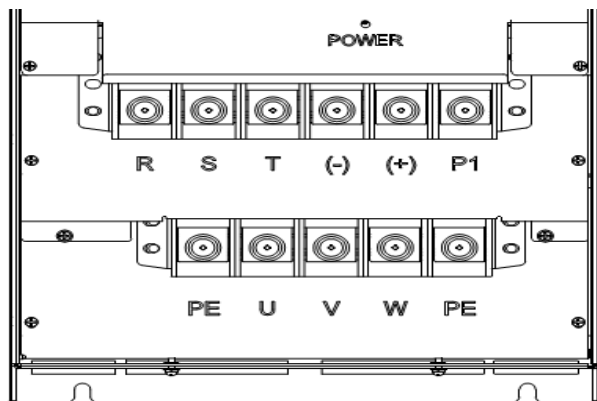
图 3-12 CT110-4T-75G~CT110-4T-110G 主回路接线端子图
