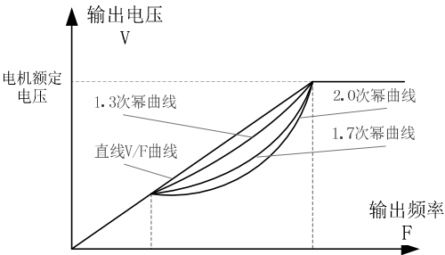
图 6-3 V/F 曲线图
