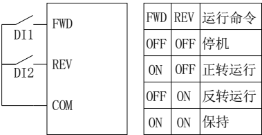
图 6-7 两线式控制 1
