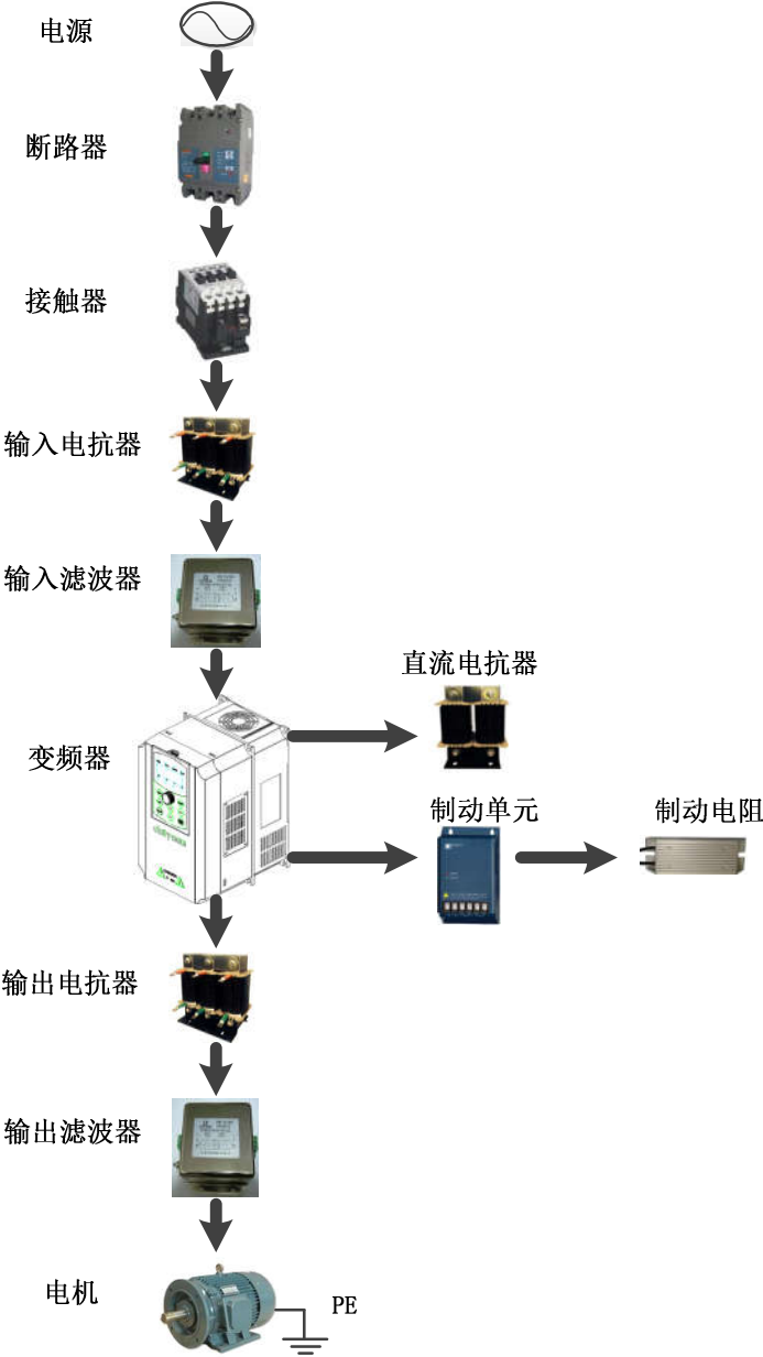
图 3-7 产品外围元器件的标准配置图
