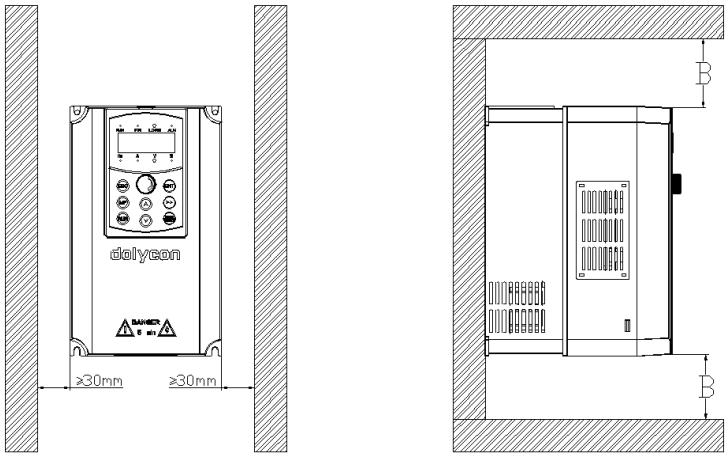
图 3-1 CT110-4T-11G/15P-B 及以下功率等级的安装方向和距离要求
