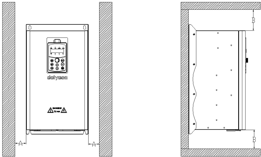
图 3-2 CT110-4T-15G/18.5P-B 及以上功率等级的安装方向和距离要求
