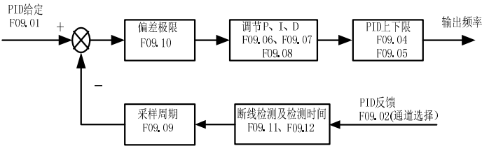
图 6-14 过程 PID 控制流程
