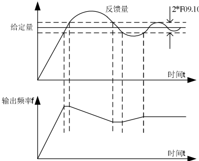
图 6-15 过程 PID 控制示例
