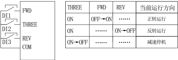
图 6-10 三线式控制 2
