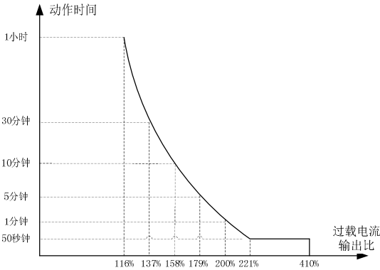
图 6-13 过载保护动作时间与电流比的关系
