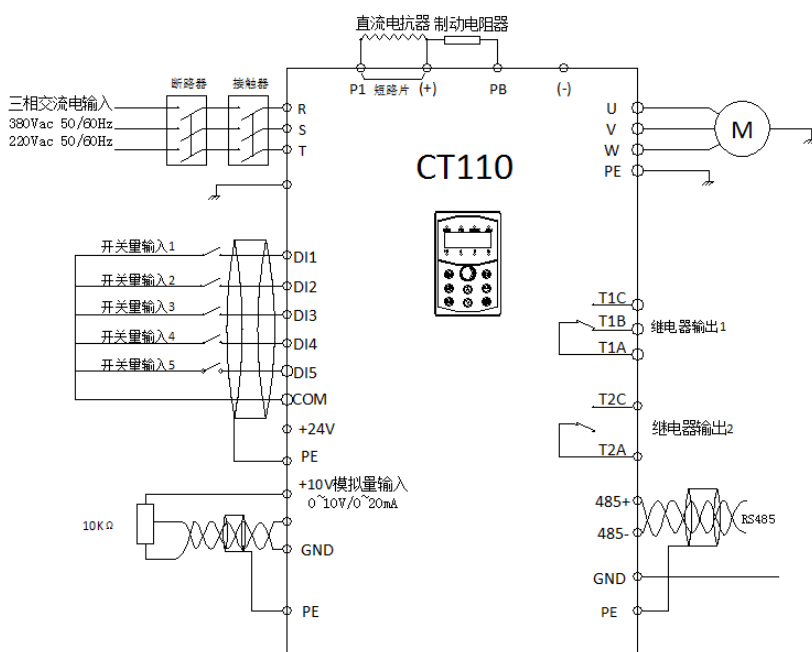
图 3-15 标准接线图
