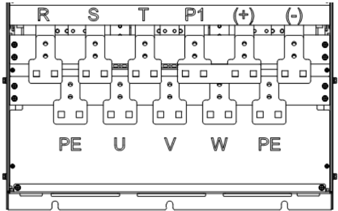
图 3-14 CT110-4T-220G~CT110-4T-315G 主回路接线端子图
