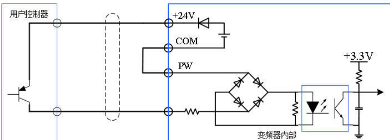
图 3-24 PNP 型拉电流接线方式
