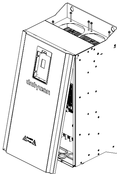
图 3-6 CT110-4T-15G/18.5P-B 及以上功率 盖板安装、拆卸图
