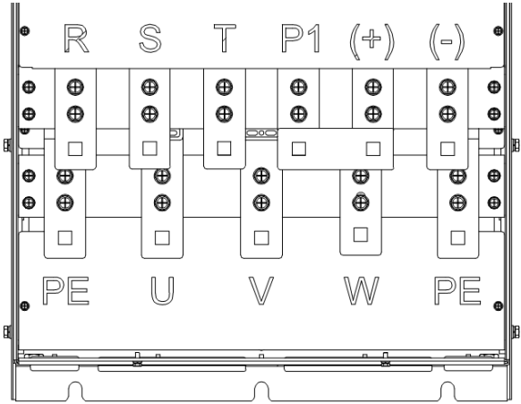
图 3-13 CT110-4T-132G~CT110-4T-200G 主回路接线端子图
