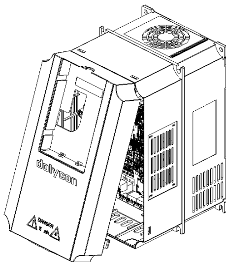
图 ( b ) 拆卸方向
