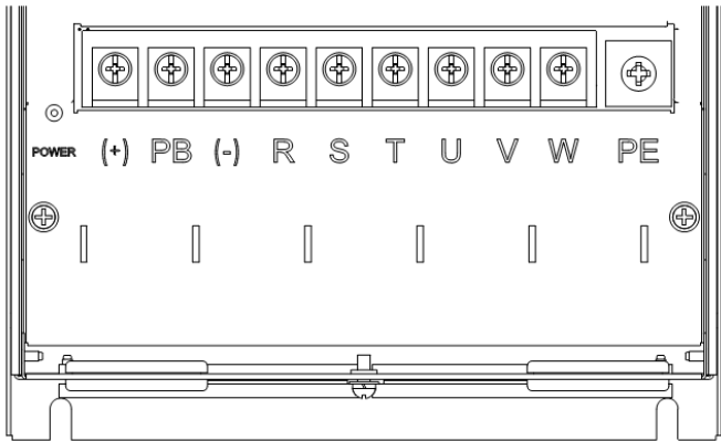
图 3-9 CT110-4T-15G-B~CT110-4T-22G-B 主回路接线端子图
