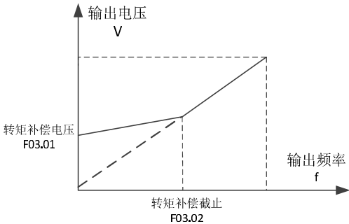
图 6-4 转矩补偿图
