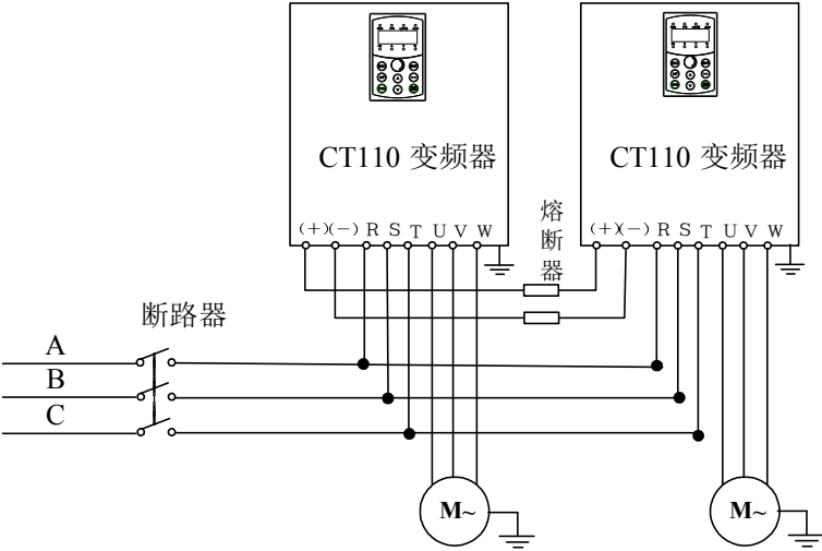
图 3-19 共直流母线的连接
