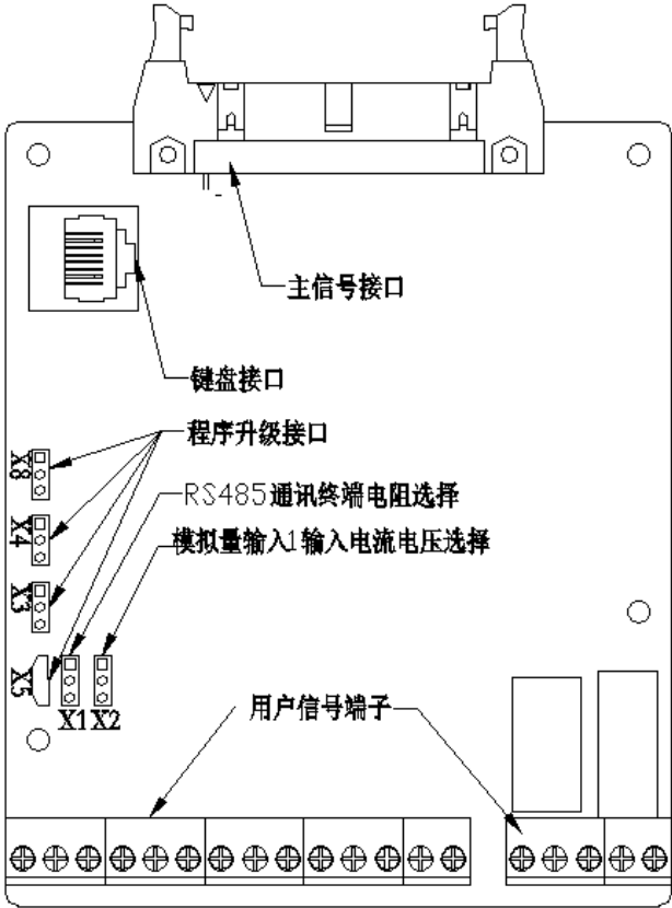
图 3-20 控制板示意图
