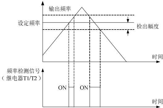
图 6-20 频率到达示意图
