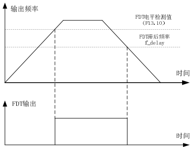
图 6-19 输出频率与 FDT 输出关系图
