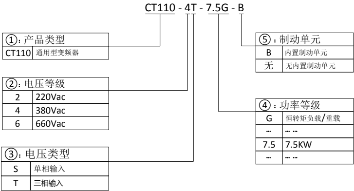
图 2-1 产品命名规则
