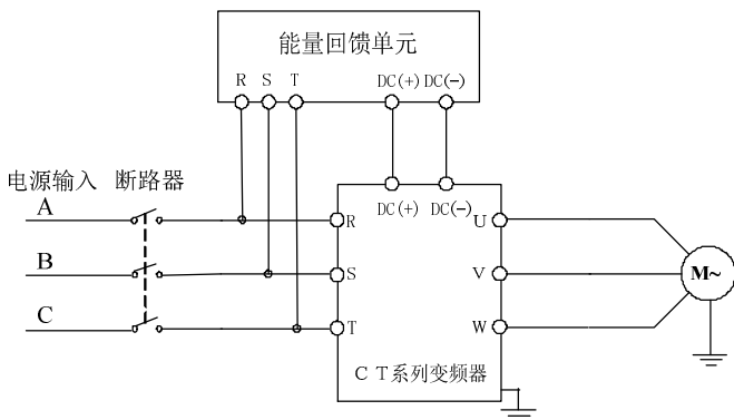
图 3-18 能量回馈单元连接图
