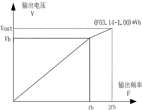
图 6-6 恒功区弱磁系数曲线图
