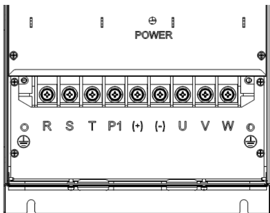
图 3-11 CT110-4T-45G~CT110-4T-55G 主回路接线端子图
