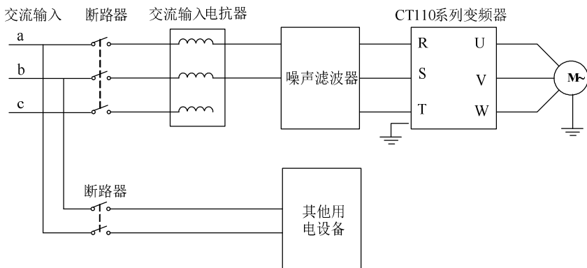
图 3-16 主回路电源侧连接图
