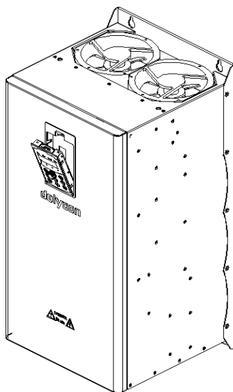
图 3-5 CT110-4T-15G/18.5P-B 及以上功率 操作面板的安装、拆卸图
