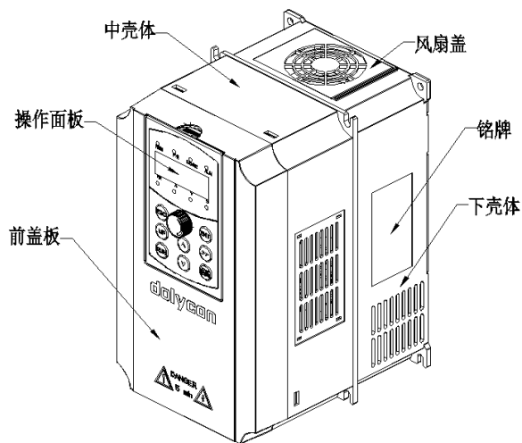
a) CT110-4T-11G/15P-B 及以下功率 (C1/ C2 机箱)
