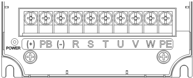
图 3-8 CT110-2S-2.2G-B、CT110-4T-11G-B 及以下功率主回路接线端子图
