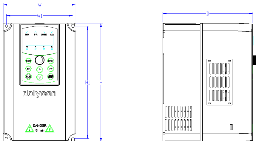
a) 适用于 CT110-2S-2.2G-B 及以下、CT110-4T-11G/15P-B 及以下
