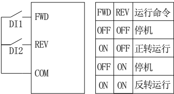
图 6-8 两线式控制 2
