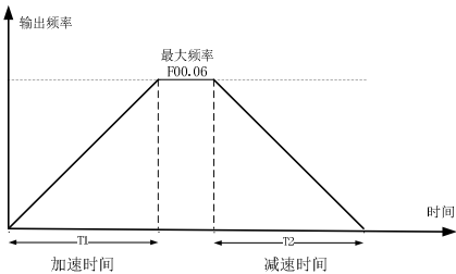
图 6-1 恒加减速曲线图
