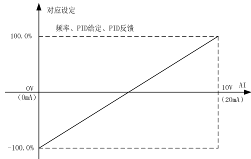
图 6-11 模拟量输入与设定值的对应关系
