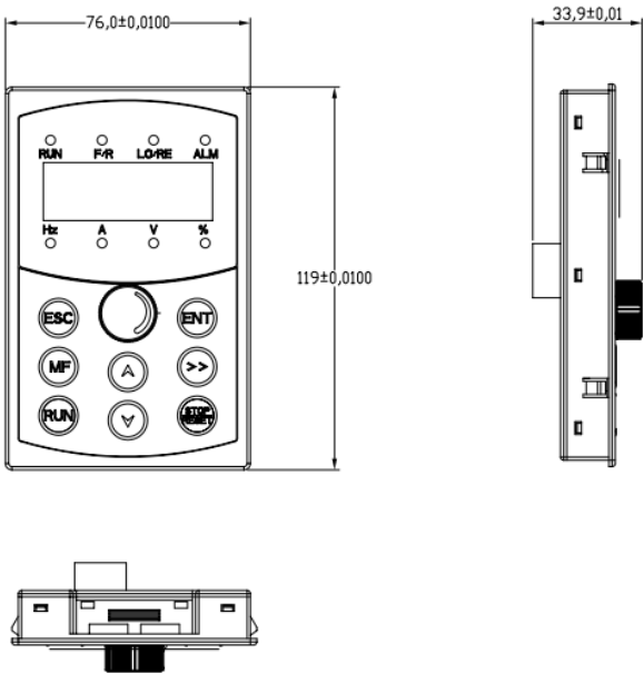
图 2-5 面板外形及尺寸图（单位 mm）
