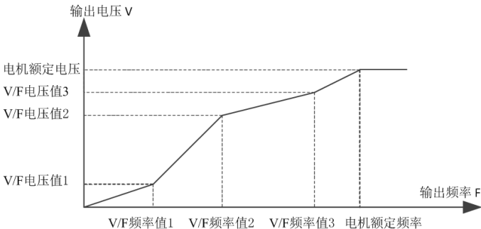
图 6-5 多段 V/F 曲线图
